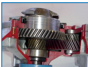
Engrenage (pignon) avec cône
